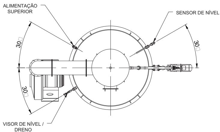
VISTA SUPERIOR ESC.: 1:50
